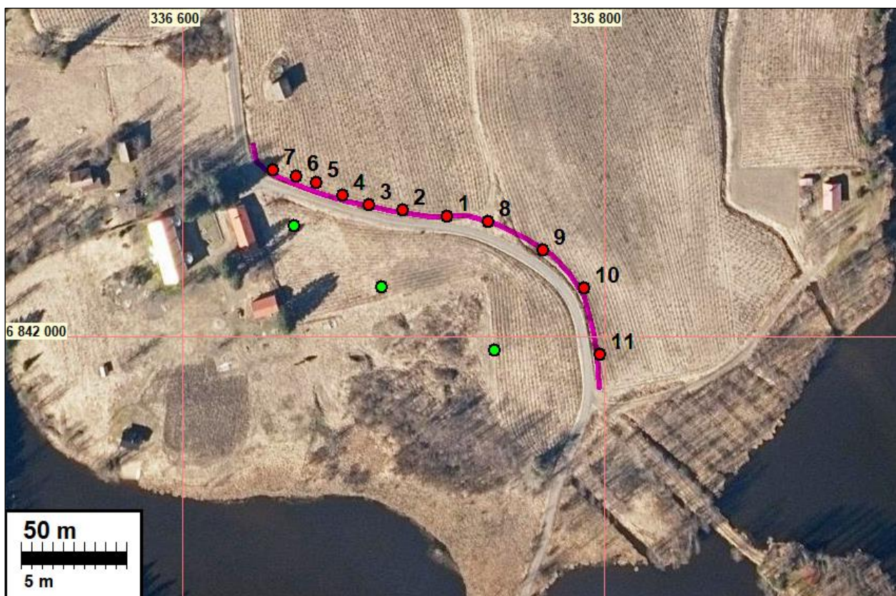
Tutkittu linja sinipunaisella, koekuopat punaisin pistein ja poistettavat pylvää vihrein pistein
